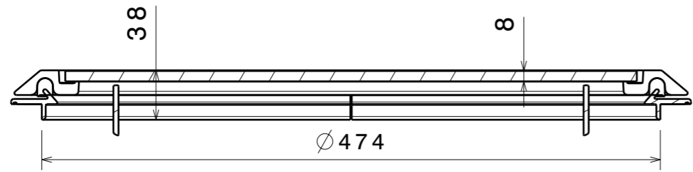
Coupe A-A Echelle : 1:4
