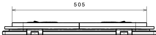
Vue de dessus Echelle : 1:7
