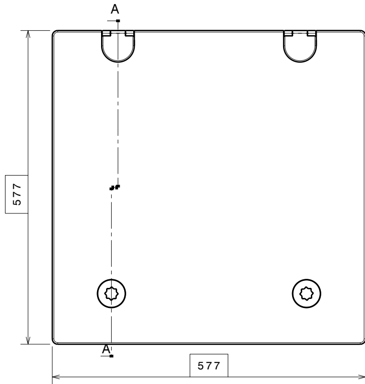
Vue de face Echelle : 1:7
