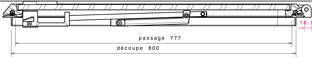
Coupe B-B Echelle : 1:5
